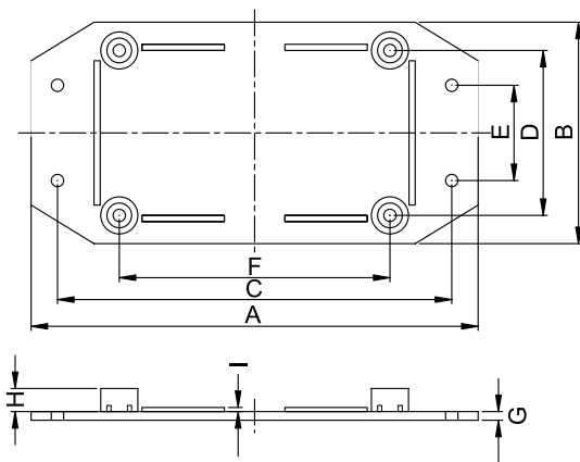
G1020BF/G1022BF/G1024BF/G1025BF
