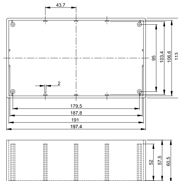
G1025B
